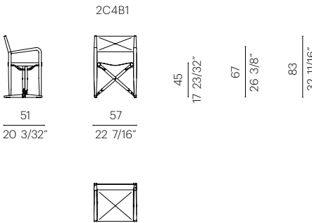
POLTRONCINA | DINING ARMCHAIR
